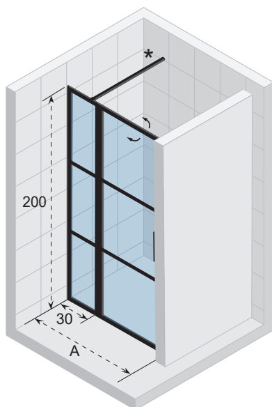
Doucheteur XL / Porte de douche XL / Duschtür XL GB104
