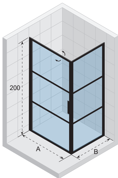
Douchecabine / Cabine de douche / Duschwand mit Eckeinstieg GB201
