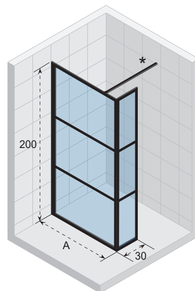
Douchewand XL / Paroi de douche XL / Duschwand XL GB402
