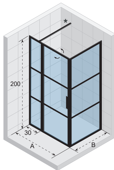
Douchecabine XL / Cabine de douche XL / Duschwand mit Eckeinstieg XL GB203
