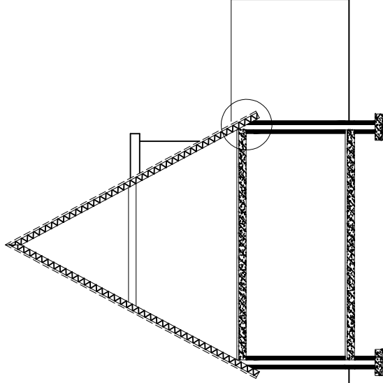
doorsnede
